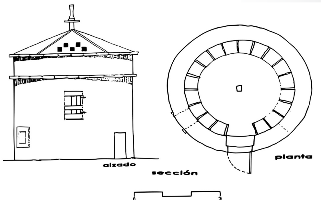
Plano de alzado do pombal. Ficha do Inventario Etnográfico da Xunta (2001). AMT
