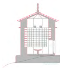
Planos do pombal. Autor: Ramón Vieites Castiñeiras
